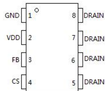
PL3325CF(SOP8)
