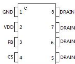
PL3325CF
