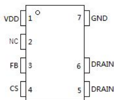
PL3325CS/D/H
