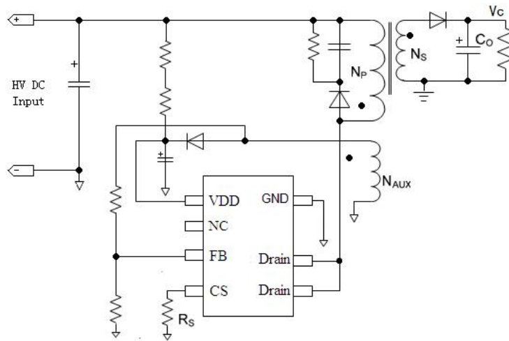
PL3325CS/D/H
